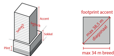
Opbouw van het accent
