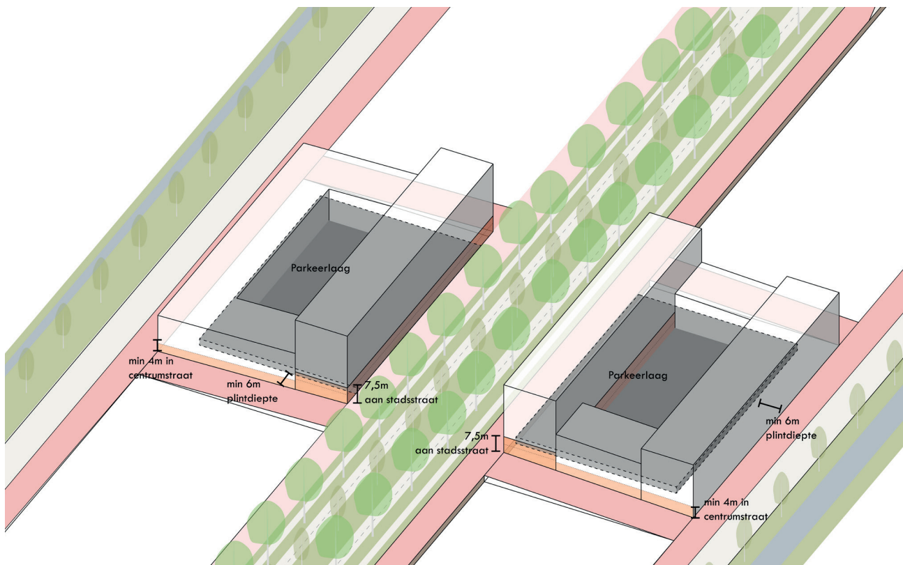
Ontwerpprincipes Plint en parkeerlaag
